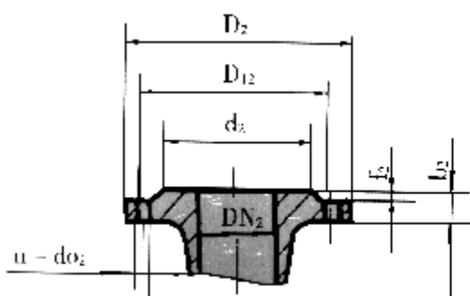
排出口法兰 DISCHARGE FLANGE
