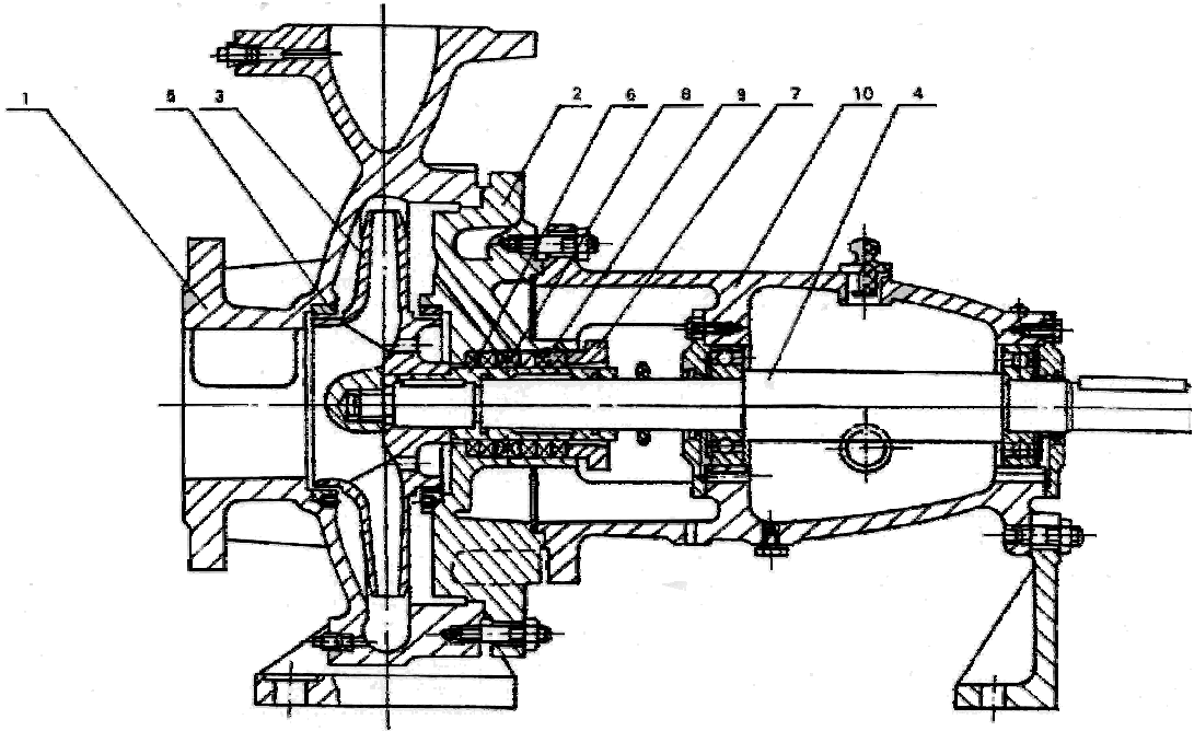
1.泵体 2.泵盖 3.叶轮 4.轴 5.密封环 6.轴套 7.填料压盖 8.填料环 9.填料 10.悬架轴承部
