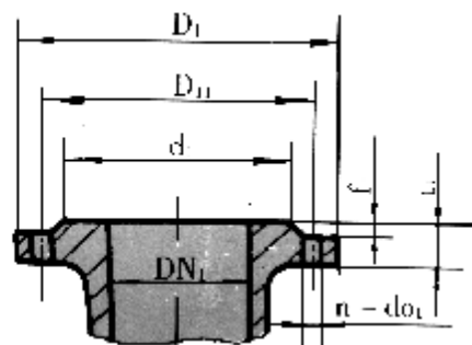
吸入口法兰 SUCTION FLANGE
